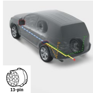
Art.-Nr. 99002-54Z00-040 E-Satz, 13-polig.
